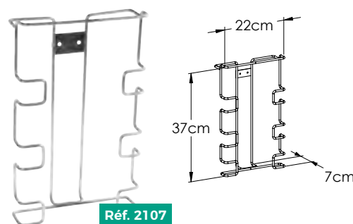
Support boîte à gants mural Inox 3 boîtes
