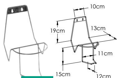
Support DOUBLE bassin de lit et urinal
