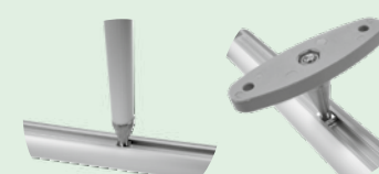
Ancrage sur rail profilé : possible à l'aide d'écrous carrés
