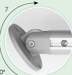
Murs inclinés, angles aigus : le raccord mural Vario RVS/WAV compense les asymétries jusqu'à 180° ainsi que les différences de longueurs jusqu'à +/- 5 mm
